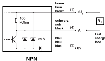
NPN
